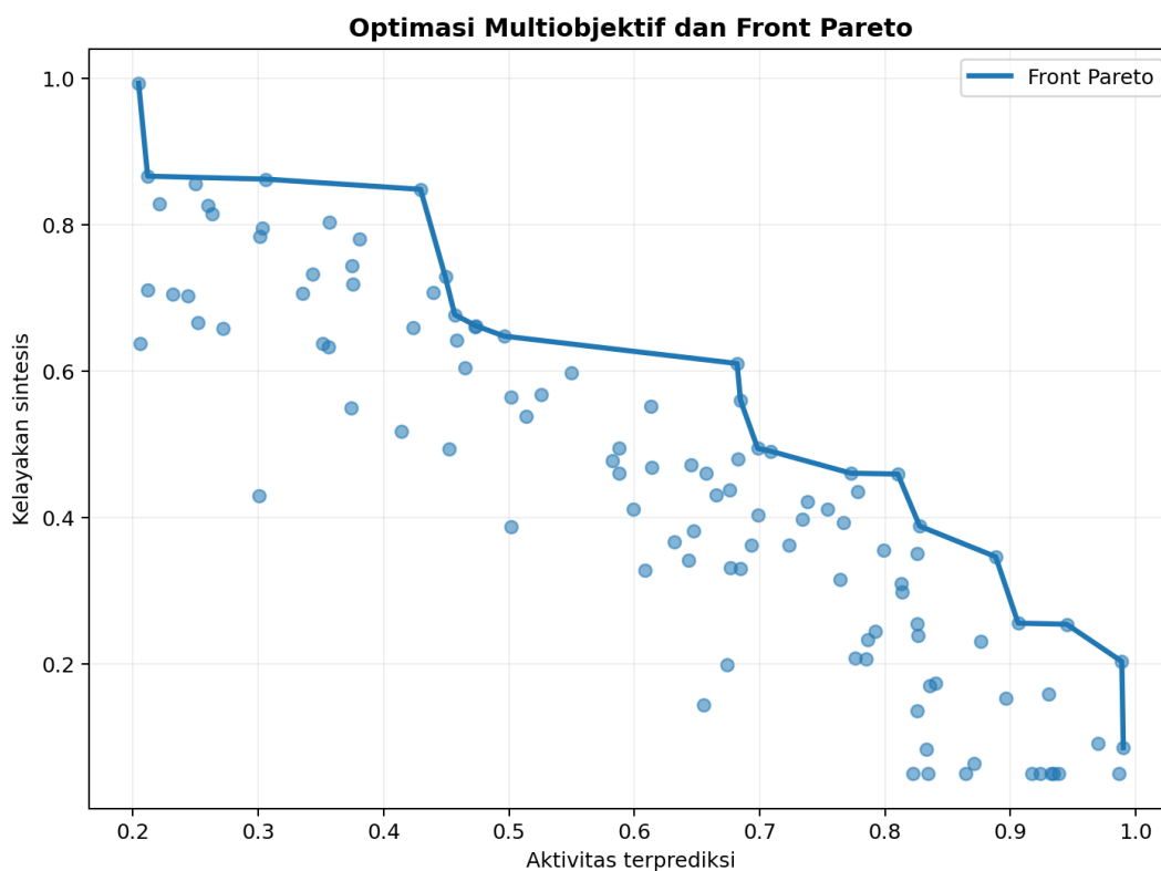
Gambar 9.2. Front Pareto menunjukkan solusi nondominan pada dua tujuan yang bertentangan.
