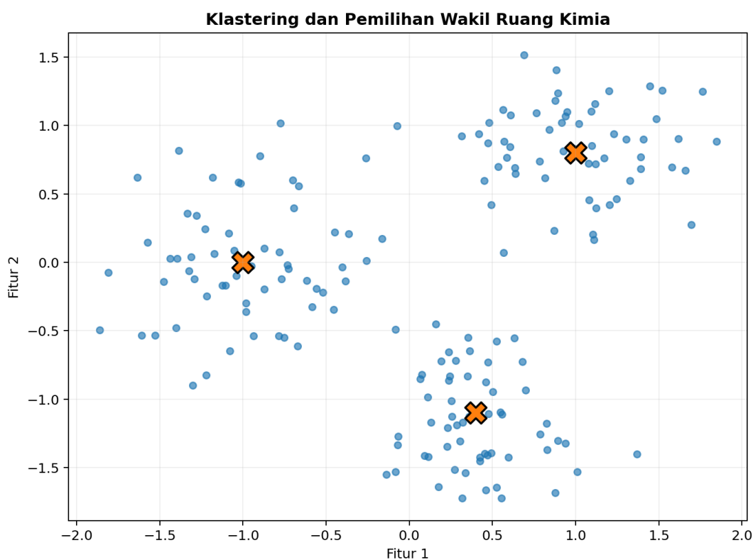
Gambar 6.2. Klastering ruang kimia dan pemilihan pusat atau medoid sebagai wakil.
