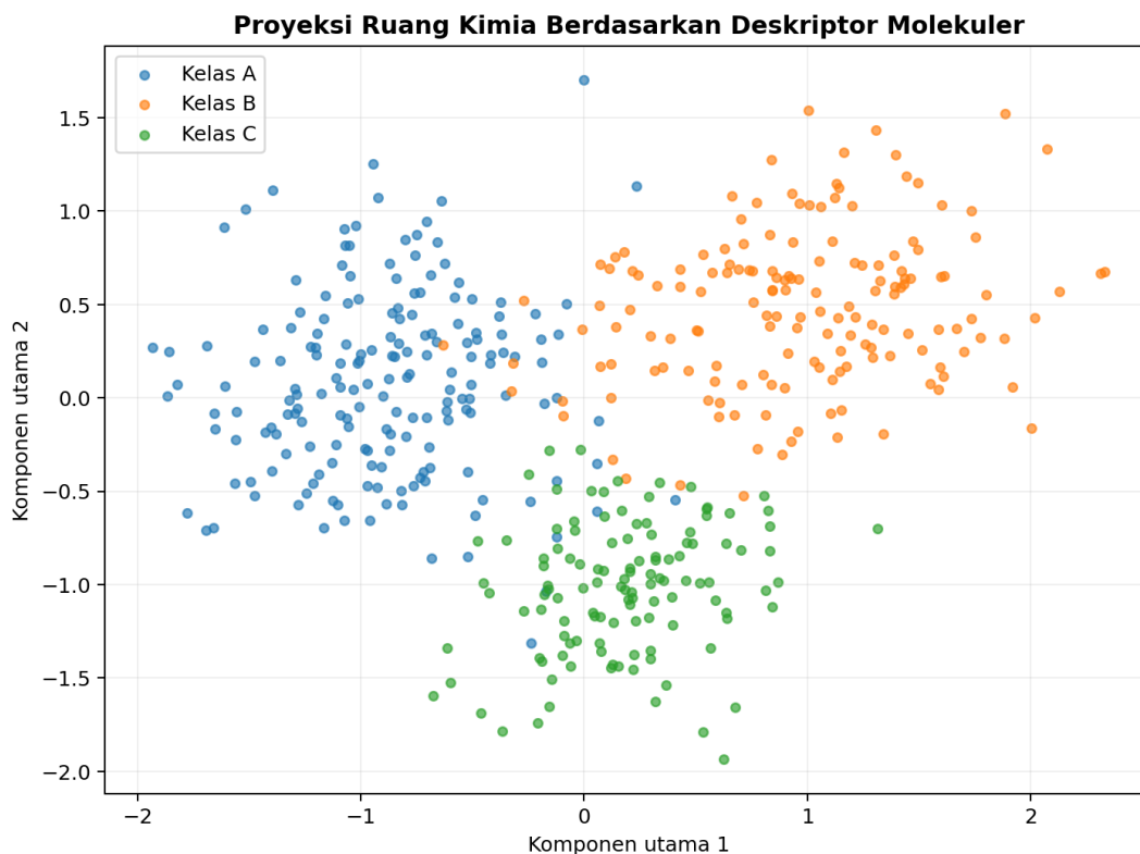
Gambar 5.1. Proyeksi dua dimensi dari ruang deskriptor berdimensi lebih tinggi.
