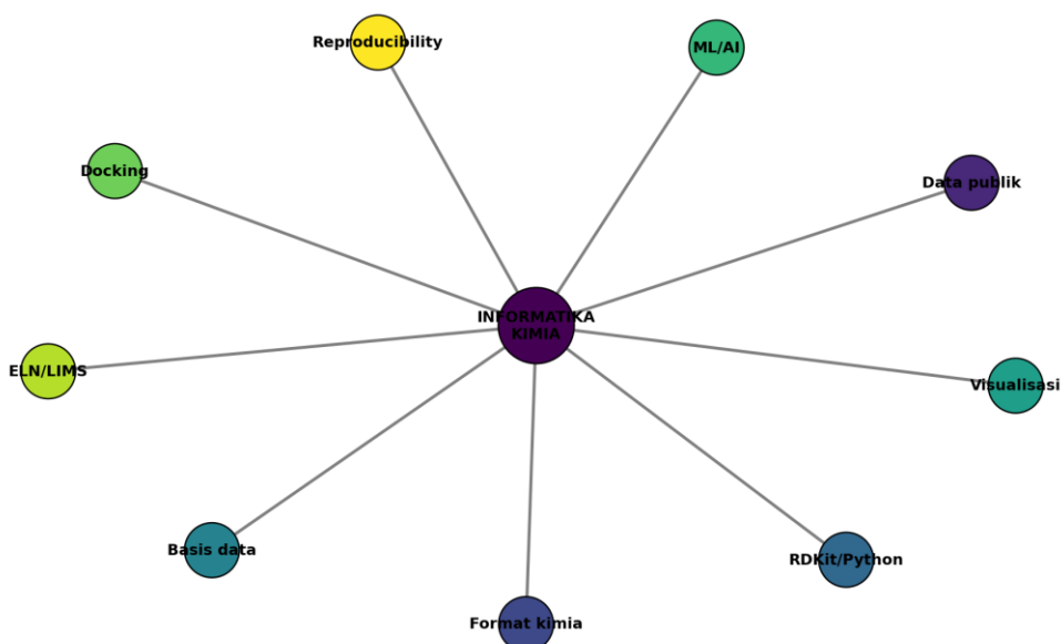
Gambar 1.2. Ekosistem disiplin, perangkat, data, dan infrastruktur informatika kimia.
