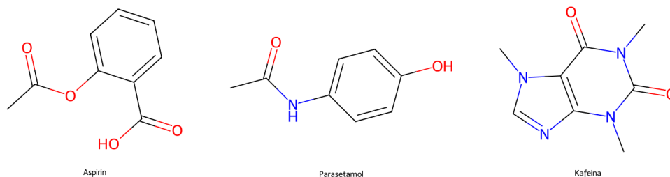
Gambar 2.1. Representasi struktur 2D aspirin, parasetamol, dan kafeina yang dibuat dengan RDKit.
