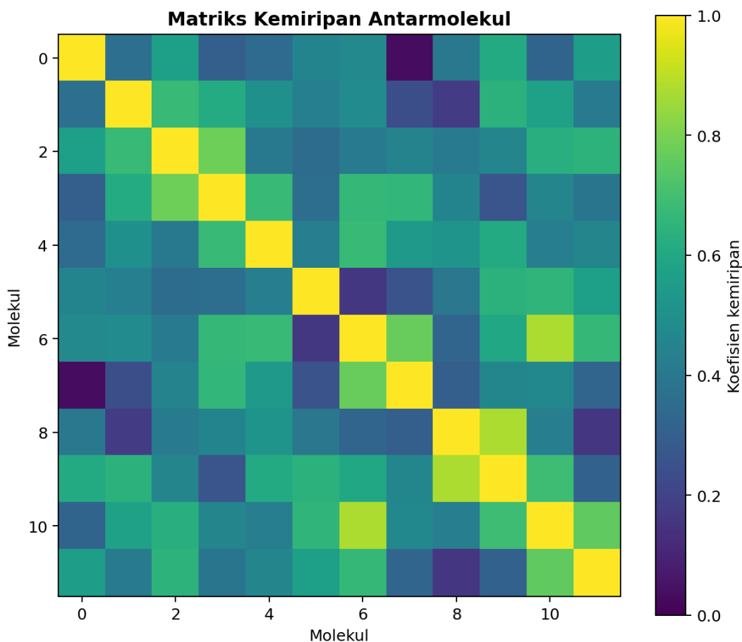
Gambar 6.1. Matriks kemiripan yang dapat menjadi dasar clustering dan pemilihan analog.
