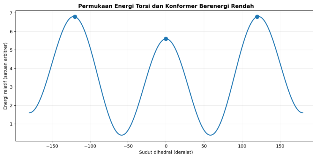
Gambar 3.1. Ilustrasi permukaan energi torsi dan beberapa minimum konformasi.
