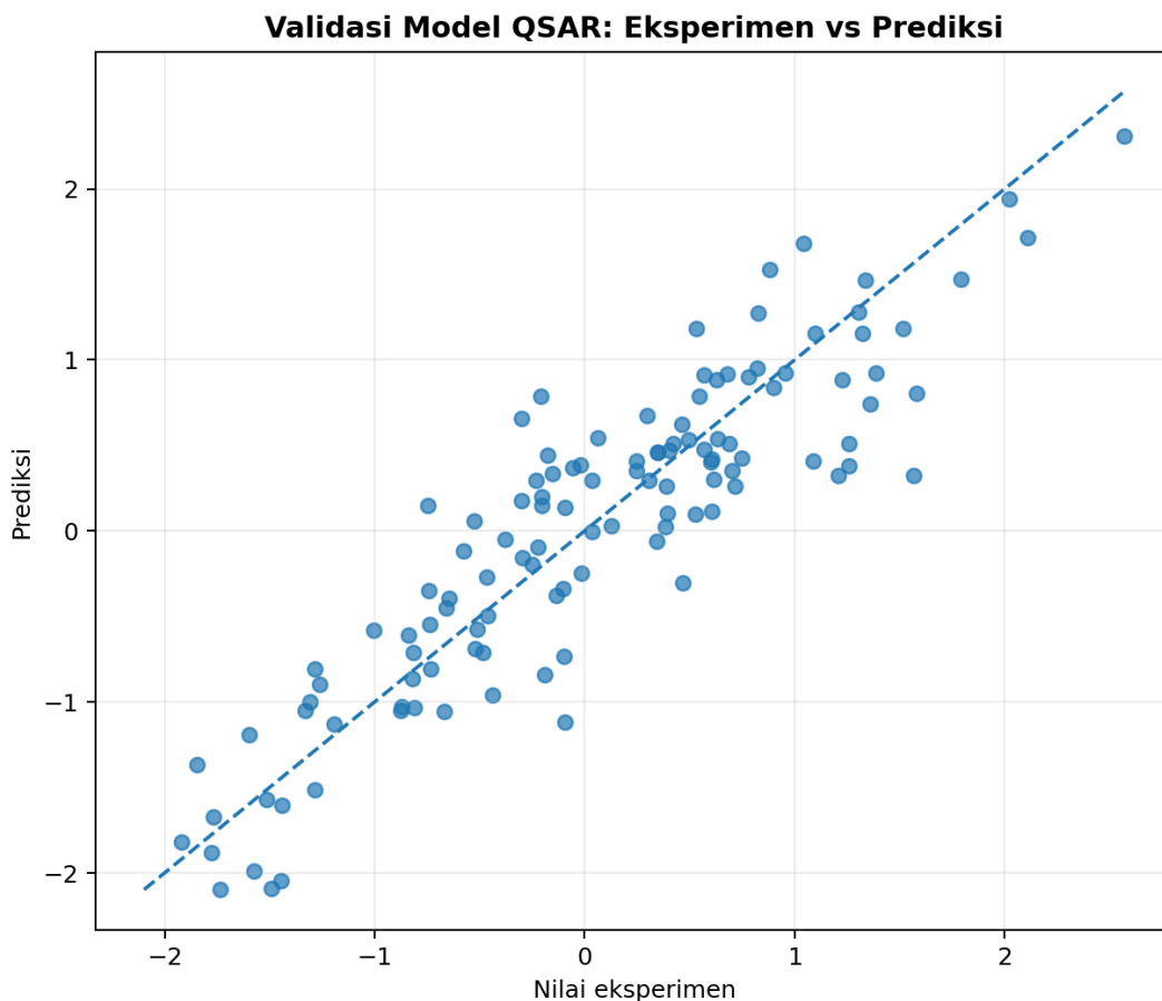
Gambar 7.2. Plot eksperimen versus prediksi sebagai salah satu diagnostik model regresi.
