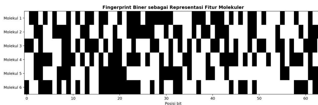
Gambar 5.2. Fingerprint biner untuk beberapa molekul; setiap baris merupakan vektor fitur.
