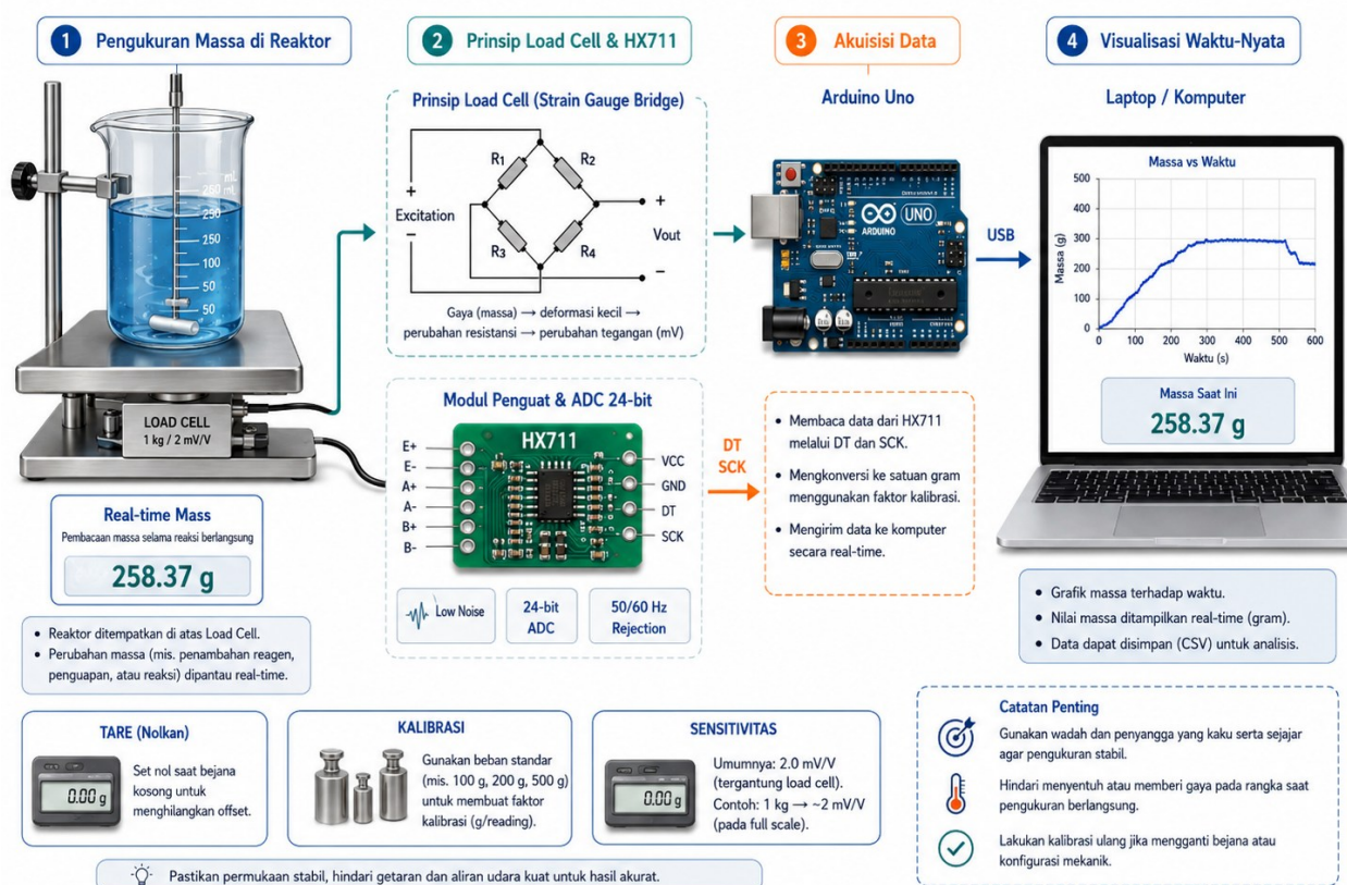
Gambar Pengembangan 12. Ilustrasi konseptual alur sensor, mikrokontroler, dan interpretasi data untuk subbab 3.3. Modul Load Cell dan HX711 untuk Pengukuran Massa Waktu-Nyata.
