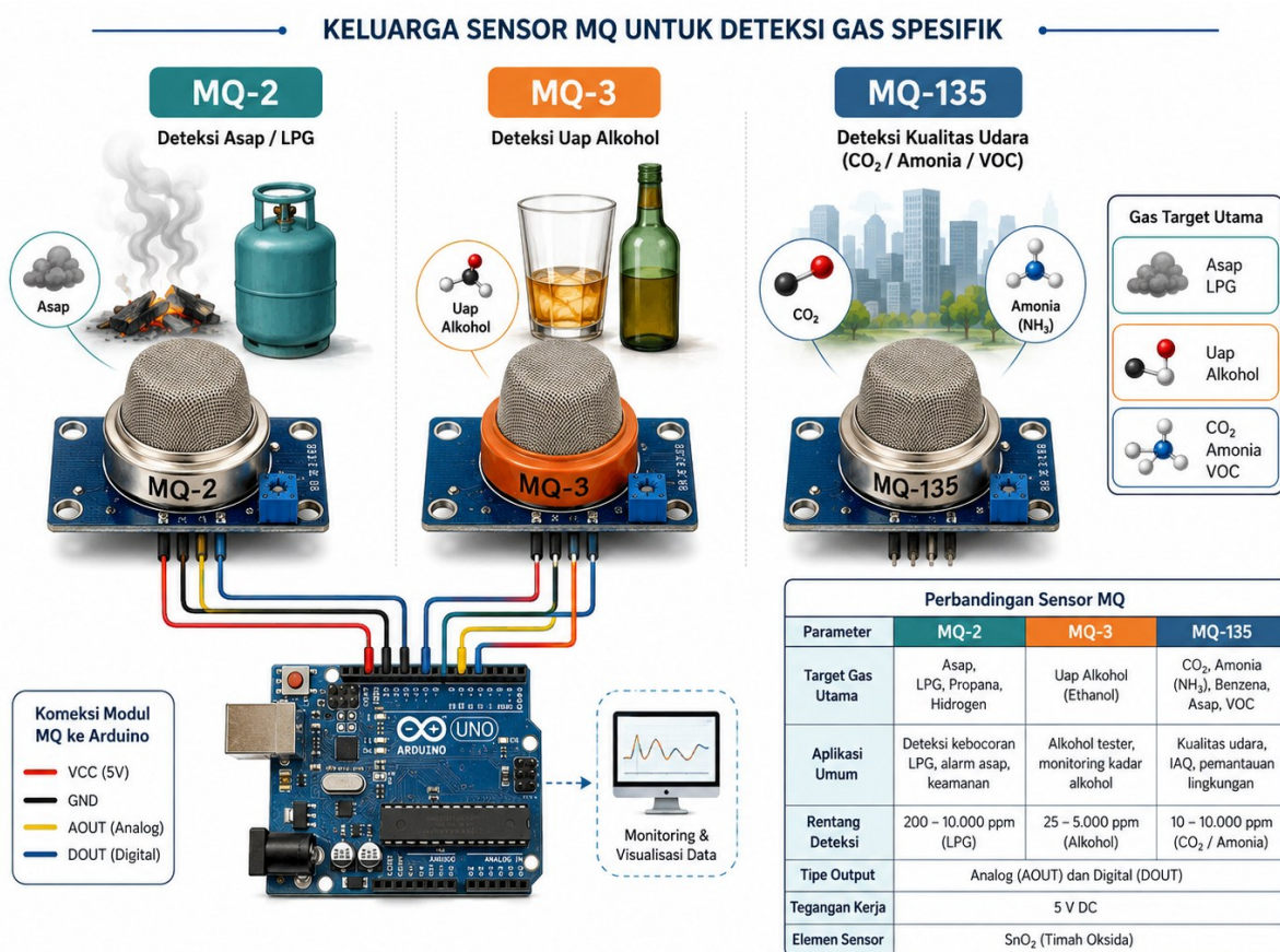
Gambar Pengembangan 26. Perbandingan Sensor MQ-2, MQ-3, dan MQ-135 untuk Deteksi Gas Spesifik
