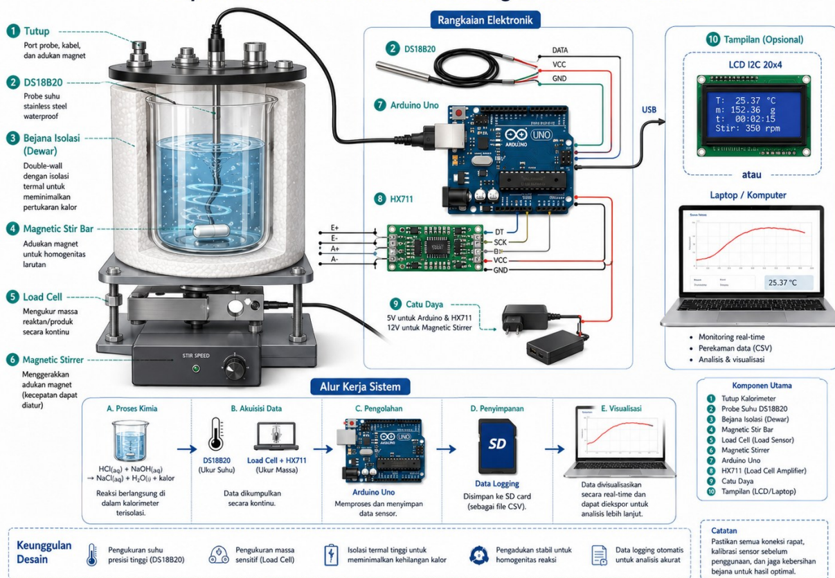
Gambar Pengembangan 13 Blueprint Alat: Merakit Kalorimeter Digital Berbasis Arduino
