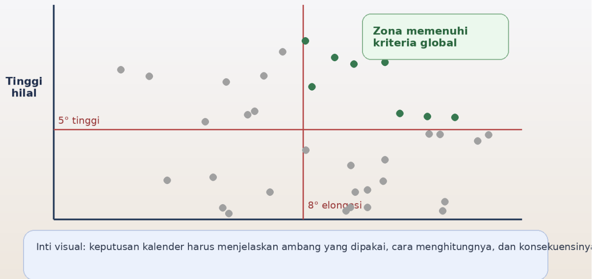
Gambar Lampiran 1.4. Ambang Kriteria Tinggi Hilal dan Elongasi
